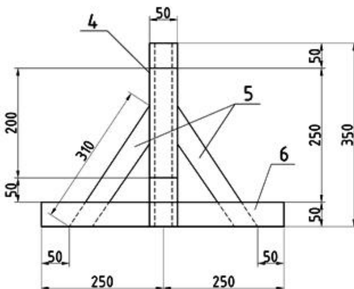
Узел "А" (подпятник)
